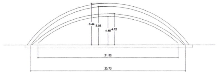
Schnitte
