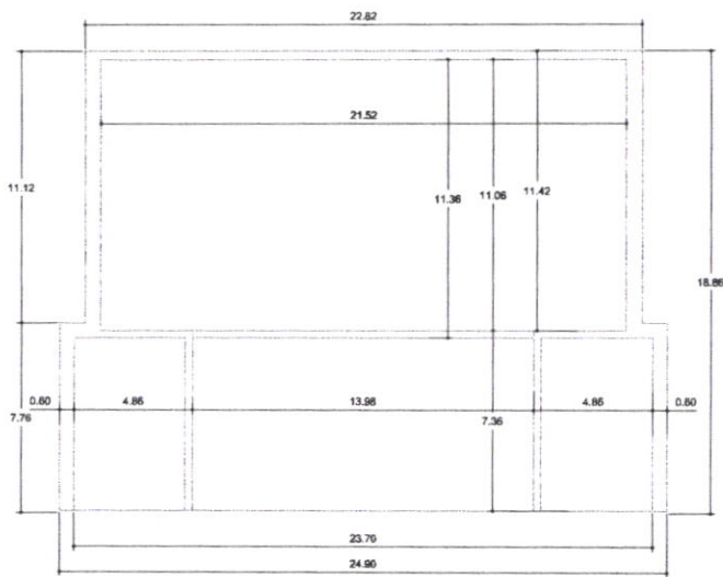
Grundriss
